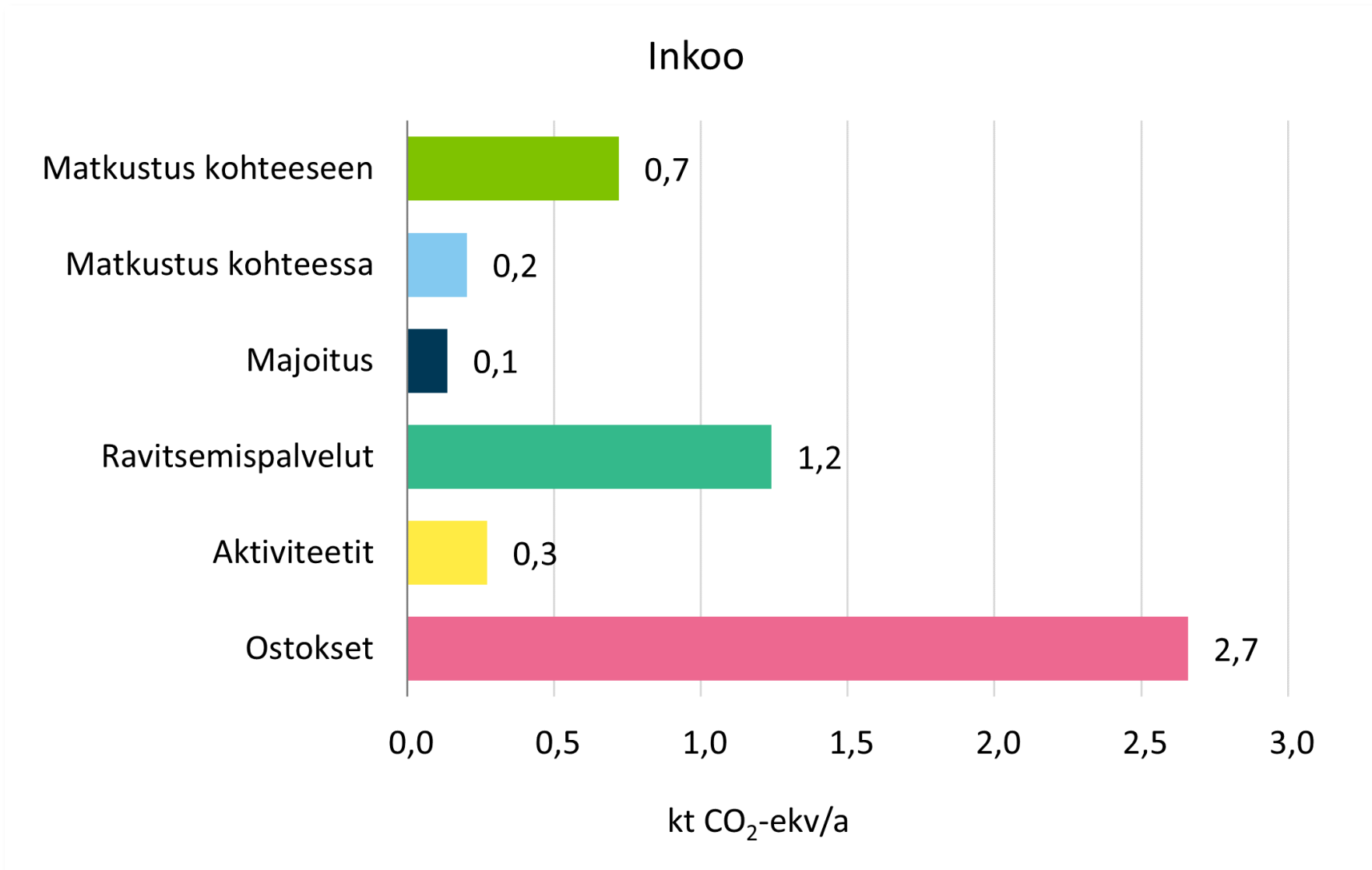
Kuva 2. Inkoon sektorikohtaiset matkailupäästöt hiilidioksidiekvivalentteina kt CO 2 -ekv. Ostosten päästöt aiheutuvat matkailusta vain osittain.
