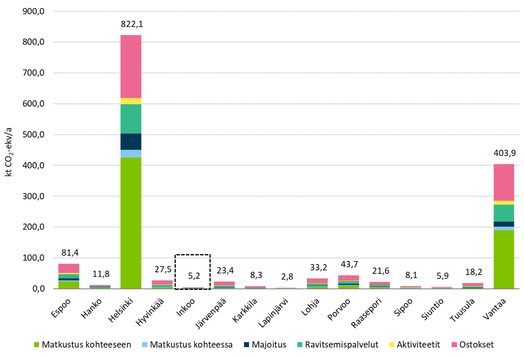
Kuva 3. Matkailun kasvihuonekaasupäästöt Inkoossa ja muissa pilottilaskennan kunnissa.
